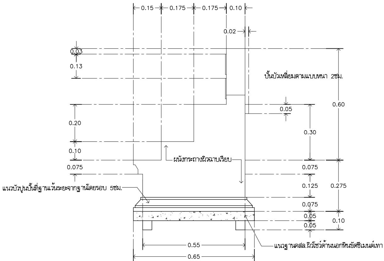
รูปด้านหลังที่ 3-3 มาตราส่วน 1:12.5
